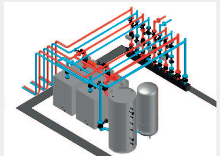
3-D CAD-Zeichnung der Heizungszentrale
